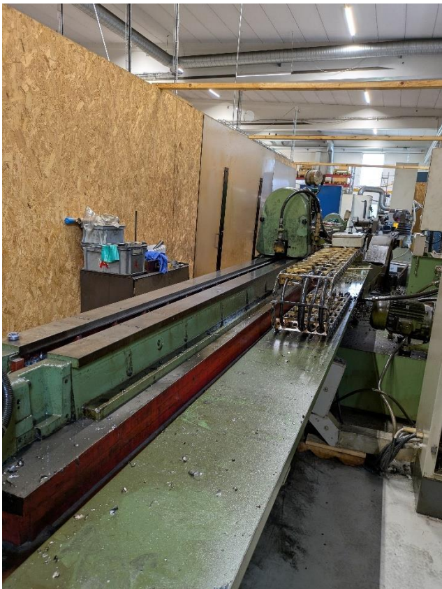
Långhålsborr TBT TE-30-2500, 80-talet.
